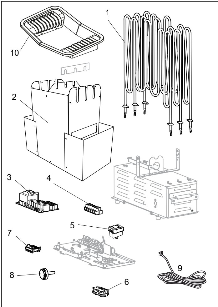
Rysunek 7. Części zamienne
